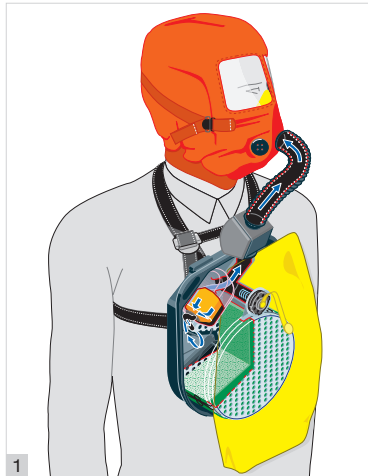
1 First inhalation cycle from starter / Erster Atemzug aus dem Starter
