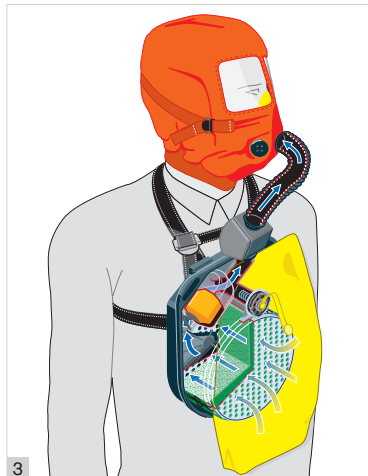
3 Inhalation cycle from breathing bag / Einatmung aus dem Atembeutel
